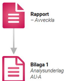
Figur 1 Dokumentstruktur Avveckla
